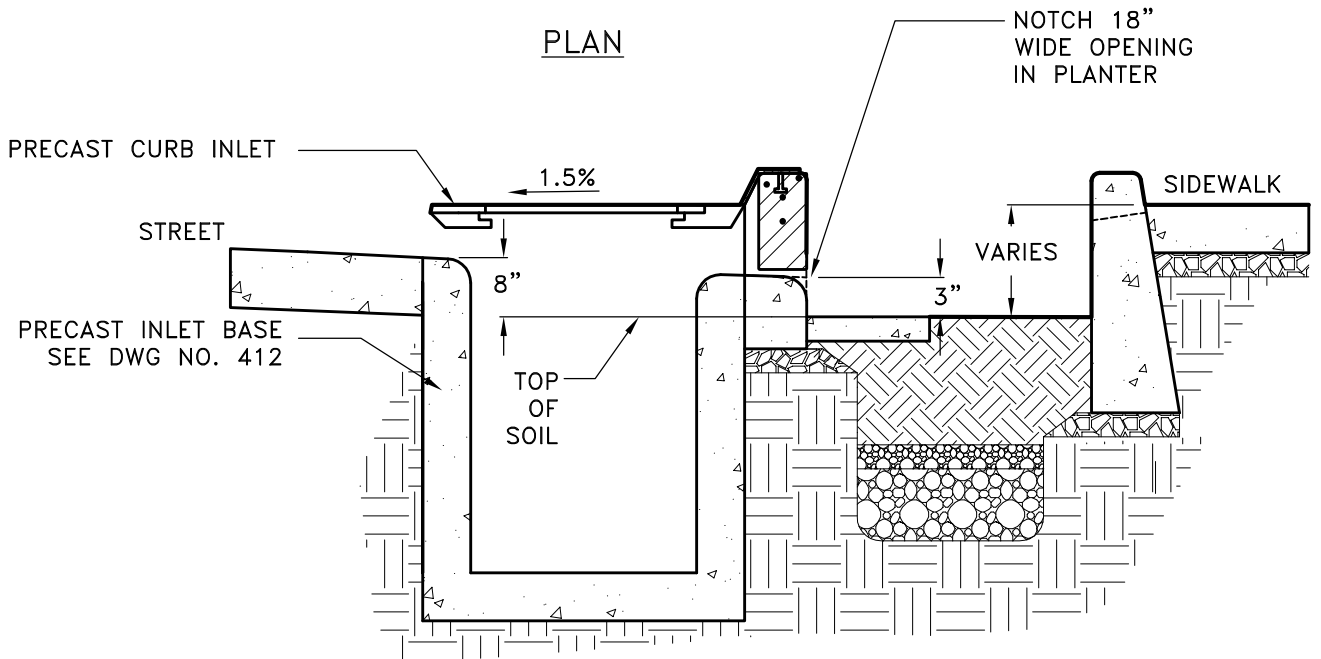
SECTION A-A
